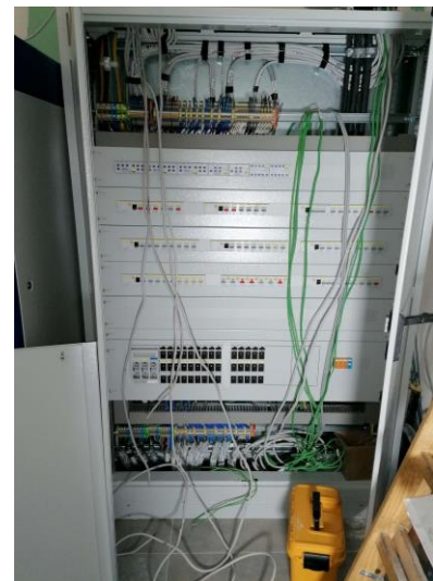
Allgemeinverteiler
